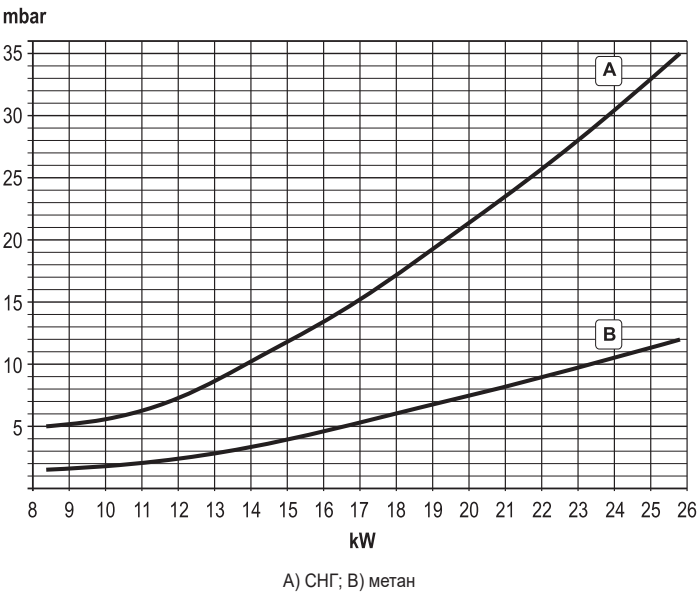
Диаграмма давление-мощность DIVAtech D HF24
