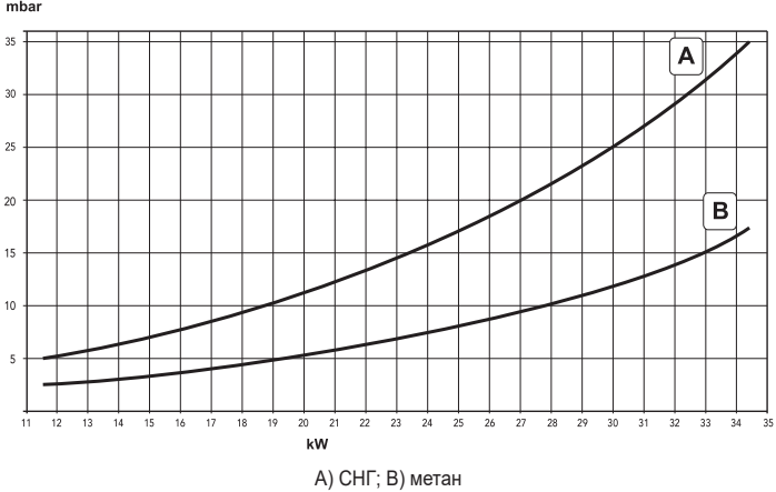
Диаграмма давление-мощность DIVAtech D HF32
