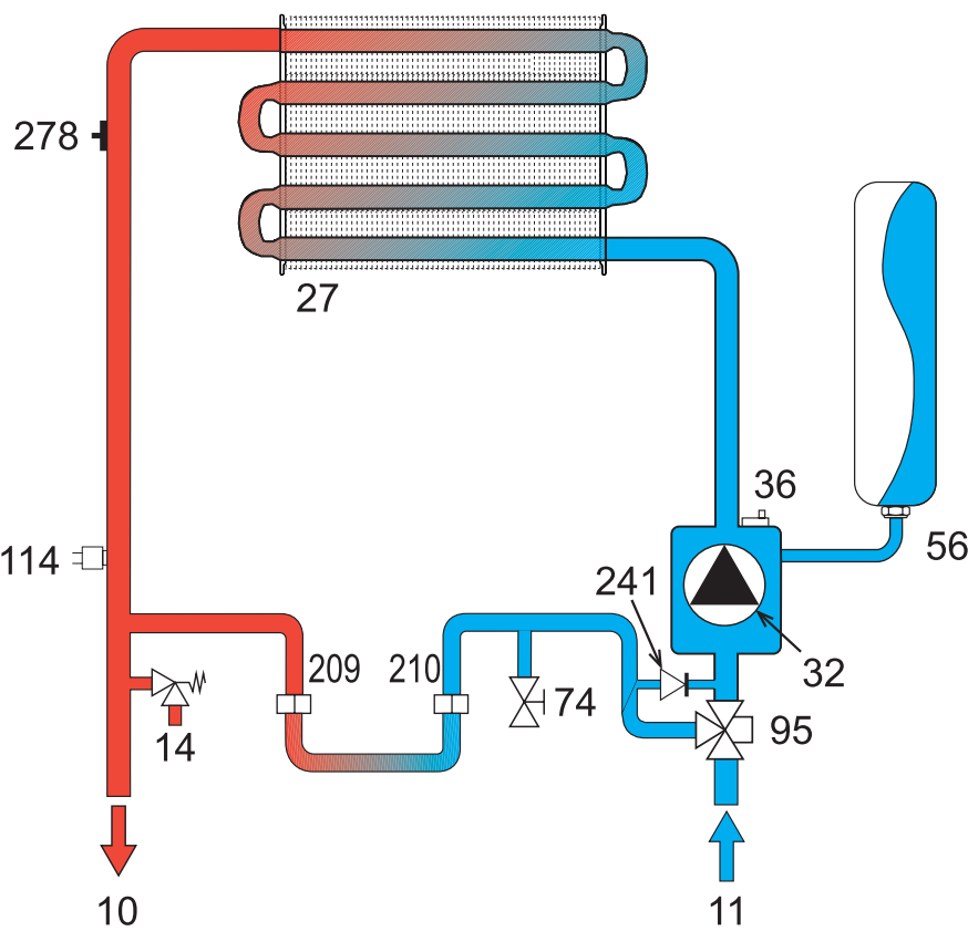
Рис. 30. Контур отопления
