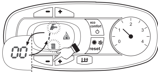
Рис. 20. Режим TEST (мощность системы отопления = 100%)
