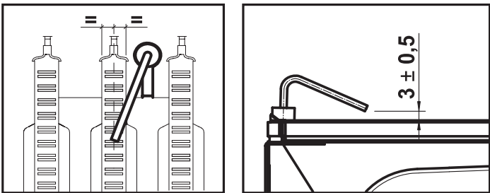
Рис. 21. Положение электрода
