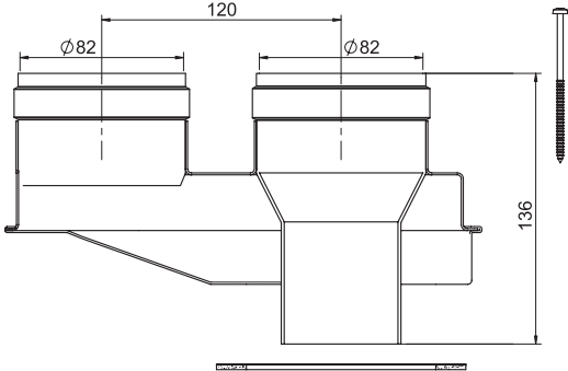
Рис 16. Адаптер для раздельных труб, код 010031X0
