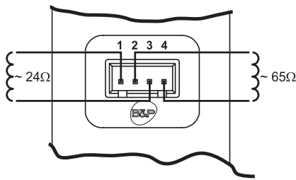
Рис. 19. Электрический разъем для подключения газового клапана TYPE SGV100 Pi макс. 65 мбар 24 В пост. тока – класс B+A
