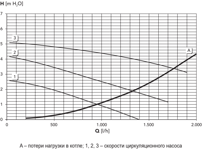
Потери нагрузки/напора циркуляционного насоса DIVAtech D HF24
