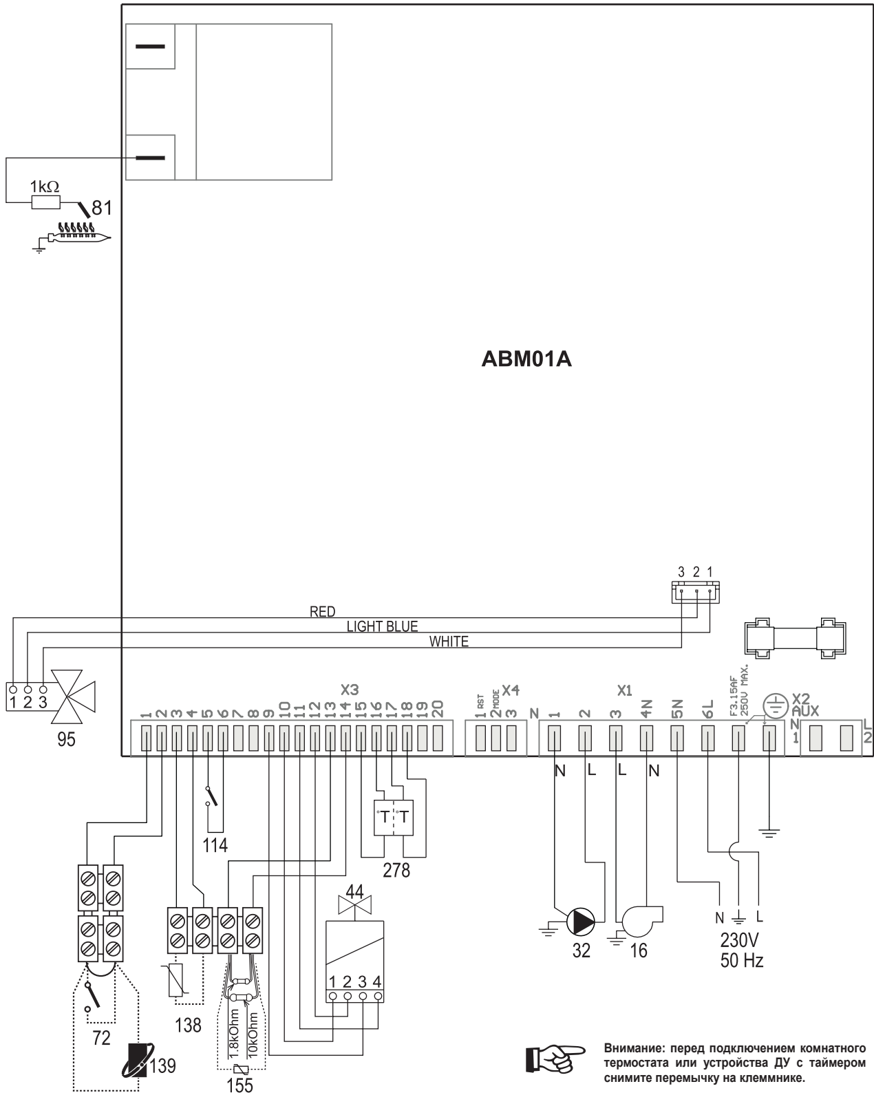
Рис. 31. Электрическая схема 16) вентилятор; 32) циркуляционный насос; 44) газовый клапан; 72) комнатный термостат (опция); 81) электрод; 95) трёхходовой кран; 114) реле давления воды; 138) уличный датчик (опция); 139) пульт дистанционного управления с таймером (опция); 155) датчик температуры воды в бойлере (опция); 278) двойной датчик (предохранительный + температуры воды в системе отопления)
