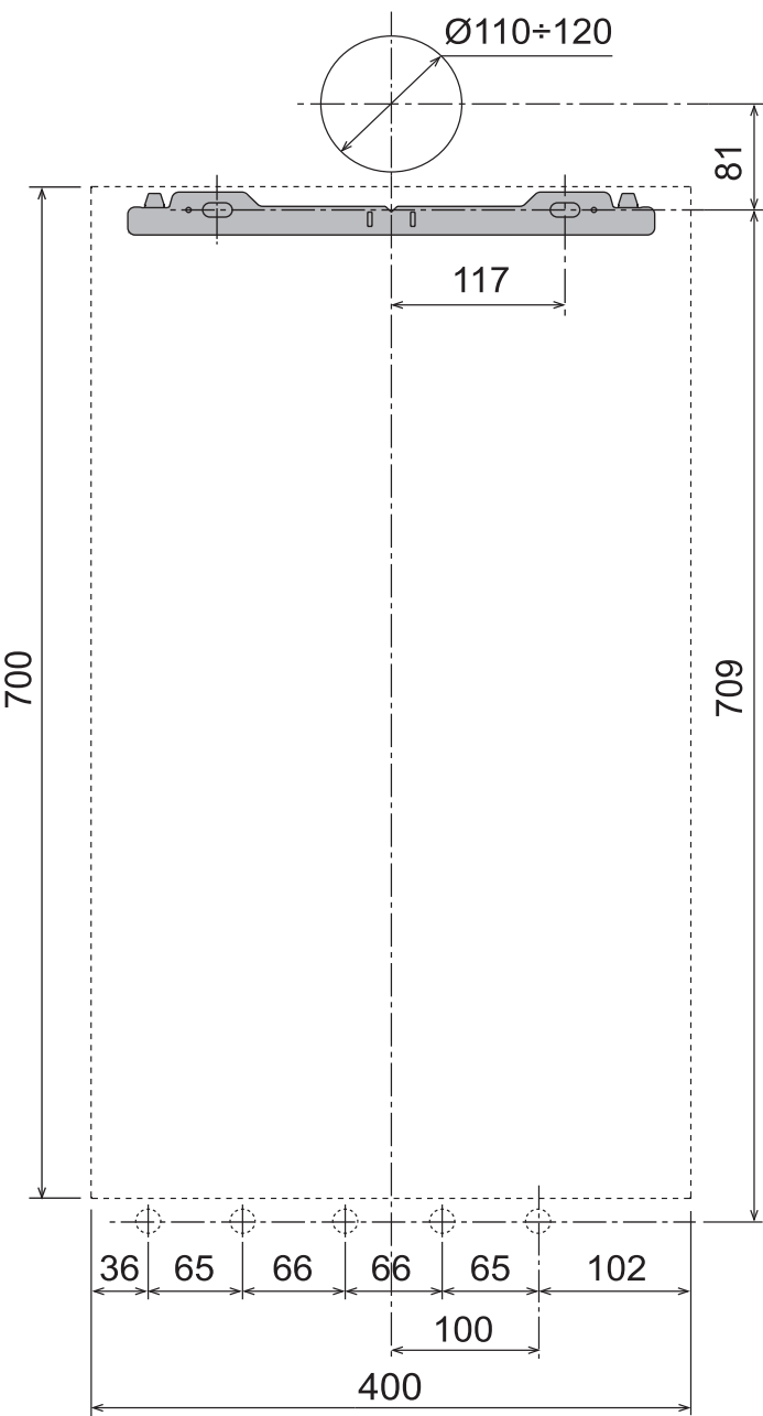
Рис. 27. Настенные отверстия
