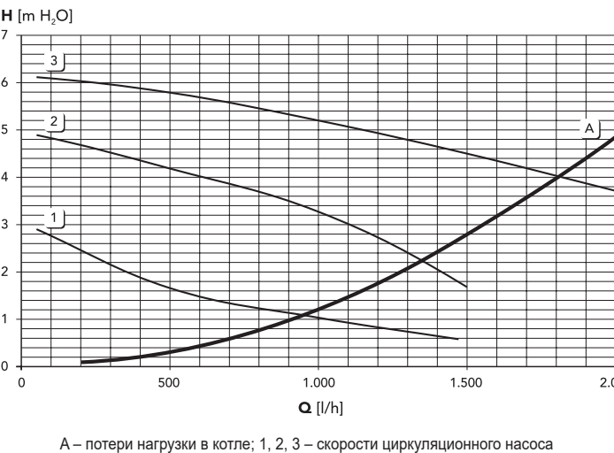
Потери нагрузки/напора циркуляционного насоса DIVAtech D HF32
